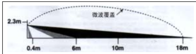
透镜侧视图
